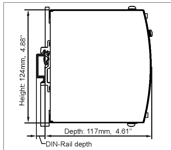
Bild 20-2 Seitenansicht
