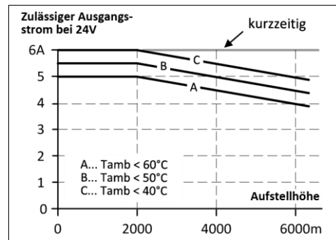
Bild 14-2 Ausgangsstrom zu Aufstellhöhe bei 24V
