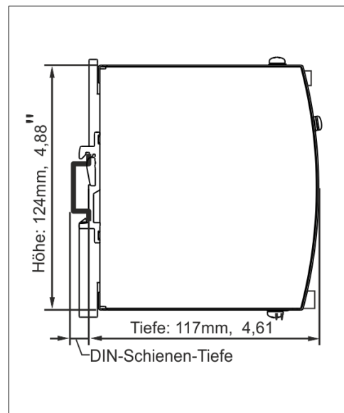
Bild 21-2 Seitenansicht
