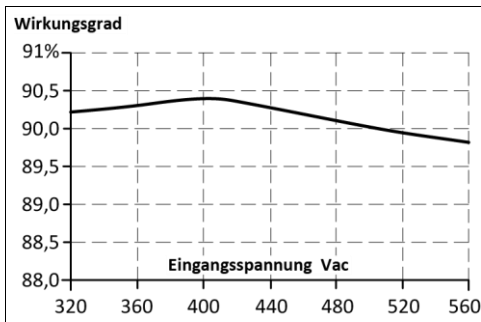
Bild 8-3 Wirkungsgrad zu Eingangsspannung bei 24V, 5A, typ.
