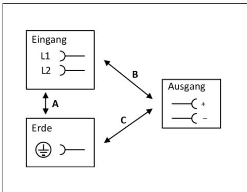
Bild 17-1 Durchschlagsfestigkeit
