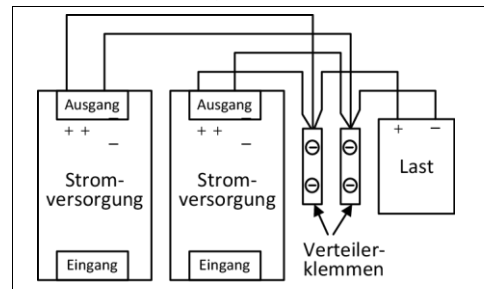
Bild 23-5 Verwendung von Verteilerklemmen
