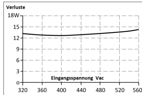
Bild 8-4 Verluste zu Eingangsspannung bei 24V, 5A, typ.
