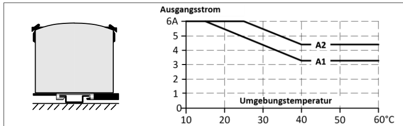
Bild 23-8 Einbaulage C (Tischmontage)
