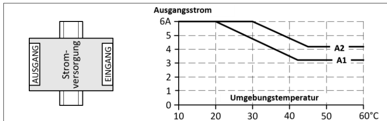
Bild 23-10 Einbaulage E (Horizontal gegen den Uhrzeigersinn)
