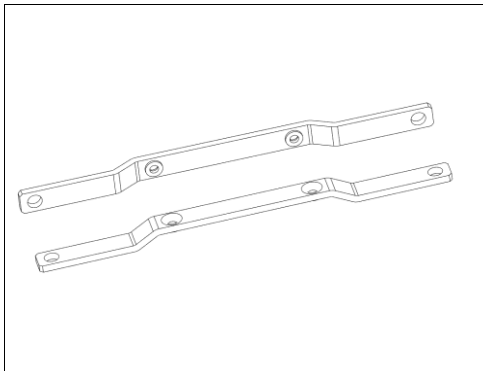
Bild 22-1 ZM1.WALL Wandmontagewinkel
