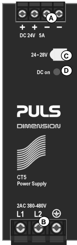
Bild 10-1 Frontseite
