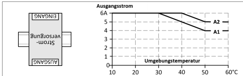
Bild 23-7 Einbaulage B (Auf dem Kopf stehend)
