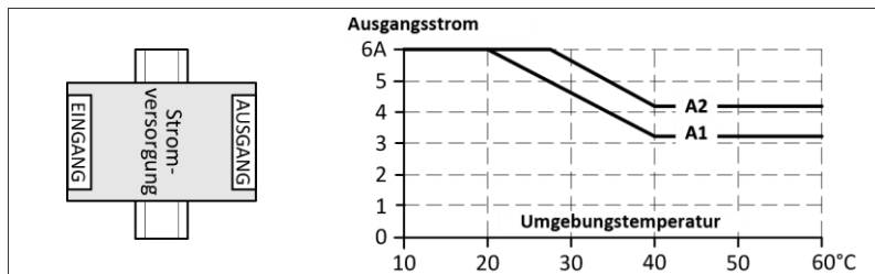
Bild 23-9 Einbaulage D (Horizontal im Uhrzeigersinn)
