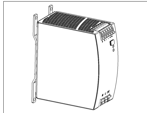
Bild 22-2 Montierter Wandmontagewinkel *)
