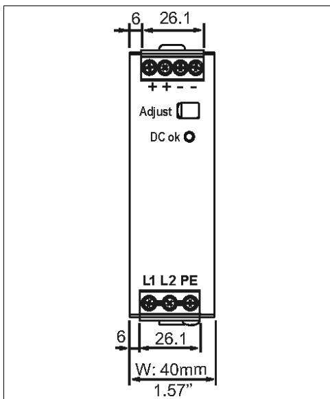
Bild 21-1 Frontansicht
