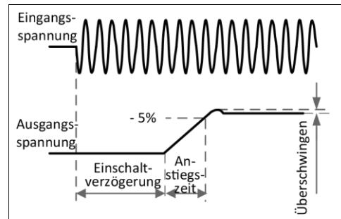
Bild 3-2 Einschaltverhalten, Definitionen
