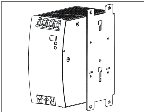
Bild 22-3 ZM12.SIDE Winkel für seitliche Montage *)
