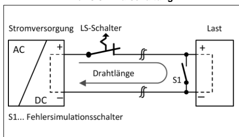
Bild 23-3 Prüfschaltung
