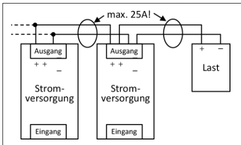
Bild 23-4 Hintereinanderschalten von Ausgängen
