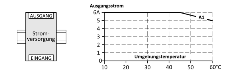
Bild 23-6 Einbaulage A (Standard- Einbaulage)
