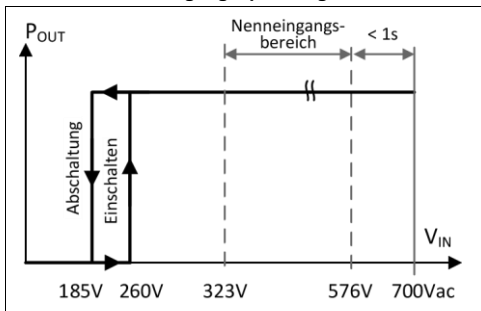
Bild 3-1 Eingangsspannungsbereich
