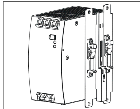
Bild 22-4 Seitliche Montage mit DIN-Schienehalterungen *)
